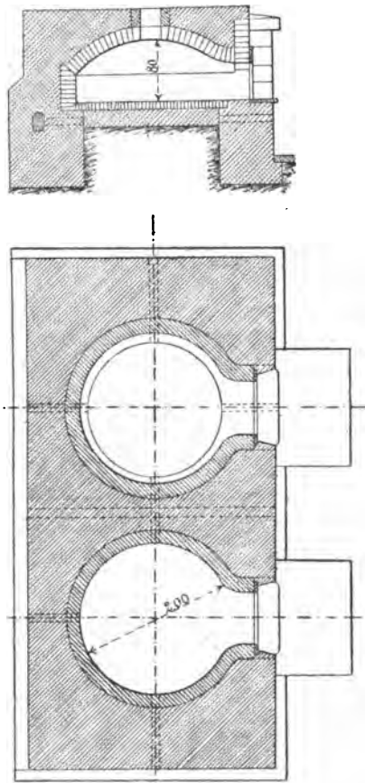
Fig. 21 et 22. — Four à boulanger.
